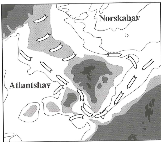
Mynd 8. Kalda rákið á 500 til 1000 m dýpi fram við Føroyum (Hansen 1993).
